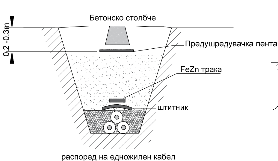
Приказ на заштита на кабел при вкрстување
