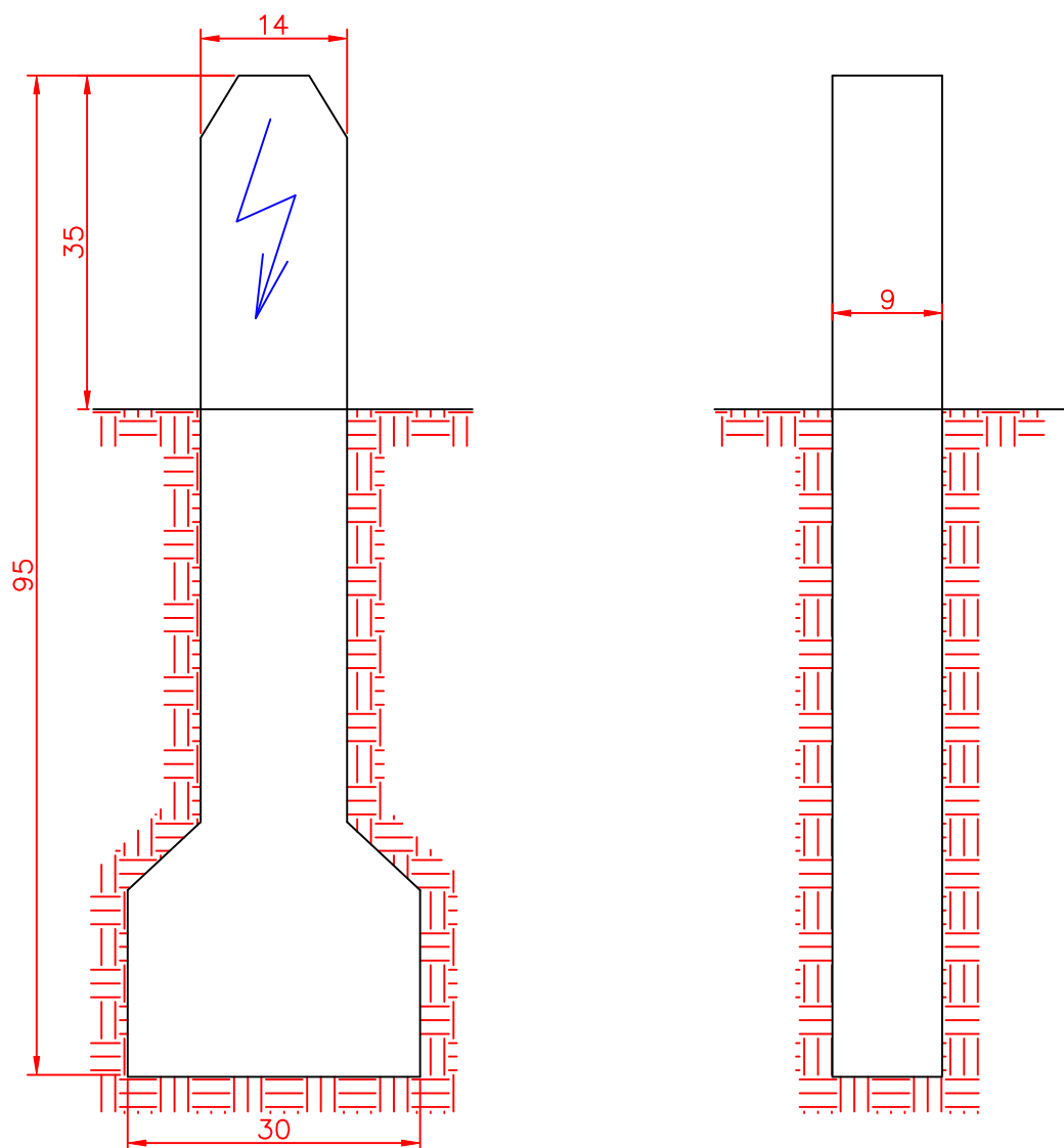
БЕТОНСКИ ОЗНАКИ ЗА БЕЛЕЖЕЊЕ НА КАБЕЛСКИ ТРАСИ
