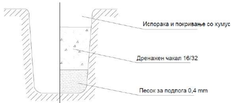
Сл. 3. Пример за ископ со три различни типа на материјал за полнење
