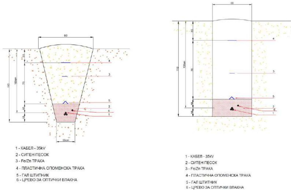
Сл. 1. Рачен ископ на ров
